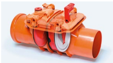
Zasawa burzowa Staufix z dwiema klapami
